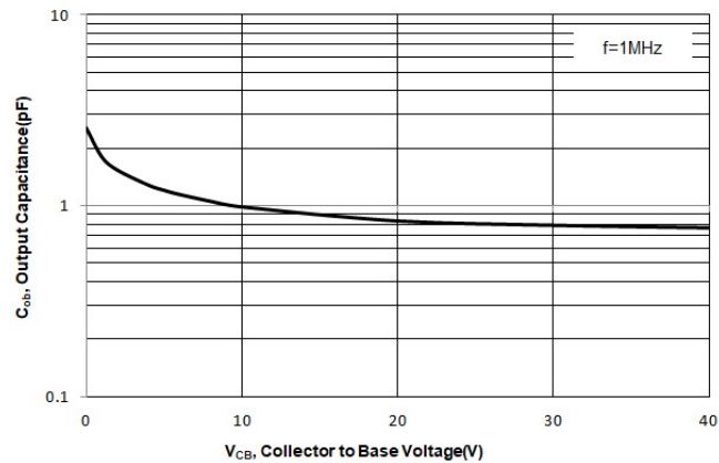
Fig. 6 Output Capacitance
